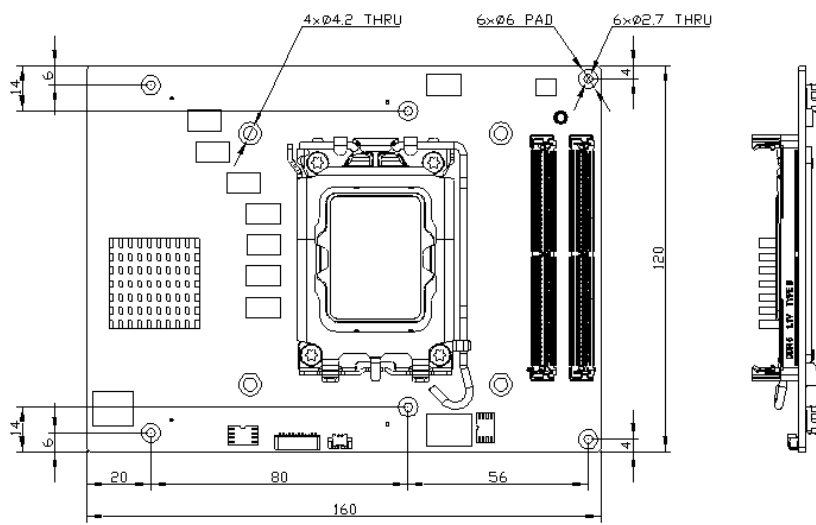
Top Side
