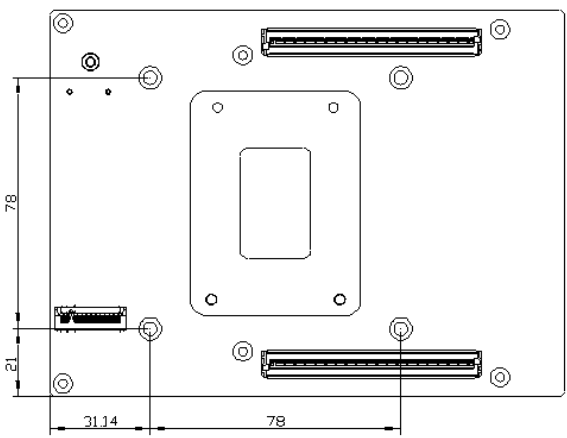
Bottom Side
