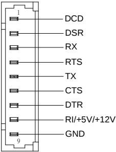
RS-232 Mode
