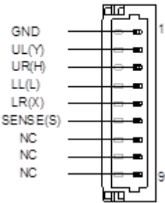
5 Wires
