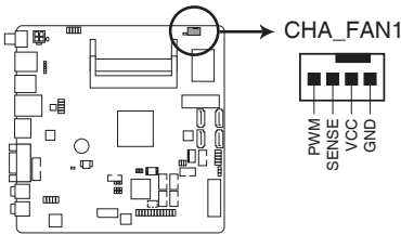
EMB-BT4 Chassis Fan connector
