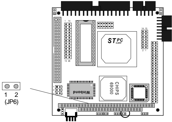
Reset switch (JP6)
