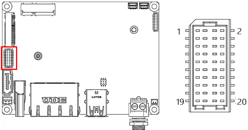
COM Port 1/Port 2 RS-232 (Default)
