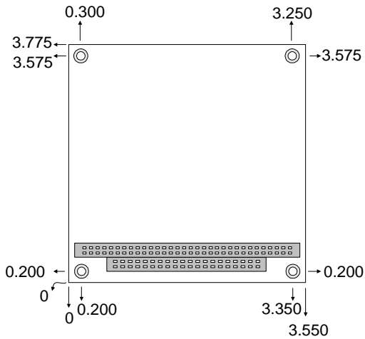
PC/104 module dimenstions (inches ? %)
