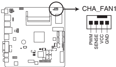
EMB-BT4 Chassis Fan connector
