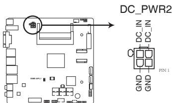
EMB-APL1 DCIN AUX power connector
