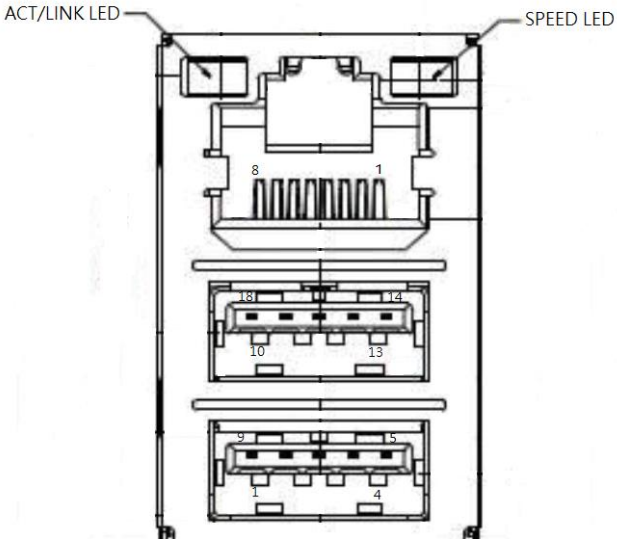
LAN (RJ-45)
