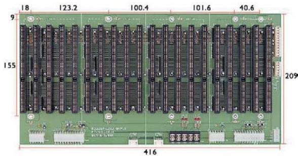
BP-220Q1-V60 Four System, 20xISA
