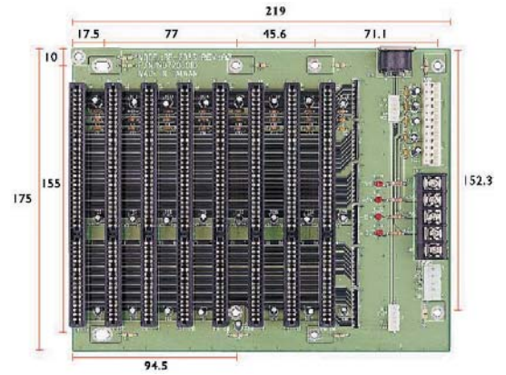
BP-208SI-A00 8xISA
