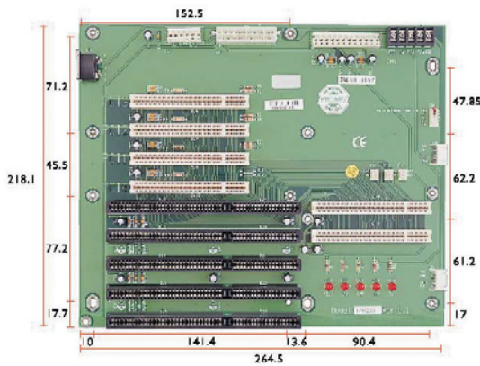
BP-209SG-P4-V61 4xPCI, 3xISA, 2xPICMG
