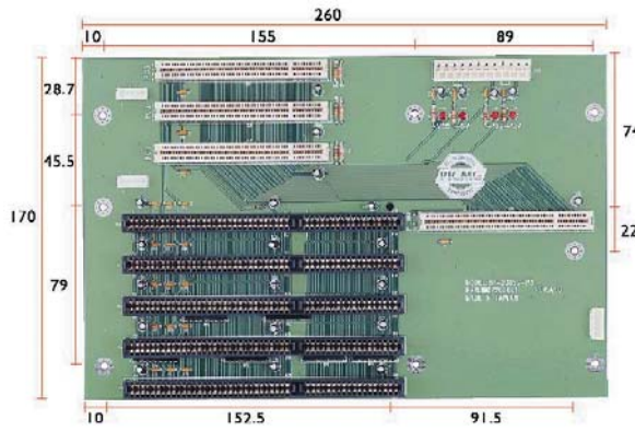
BP-208SG-P3-A10 3xPCI, 4xISA, 1xPICMG
