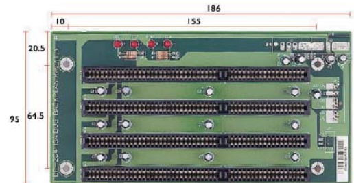
BP-204SI-A13 4xISA
