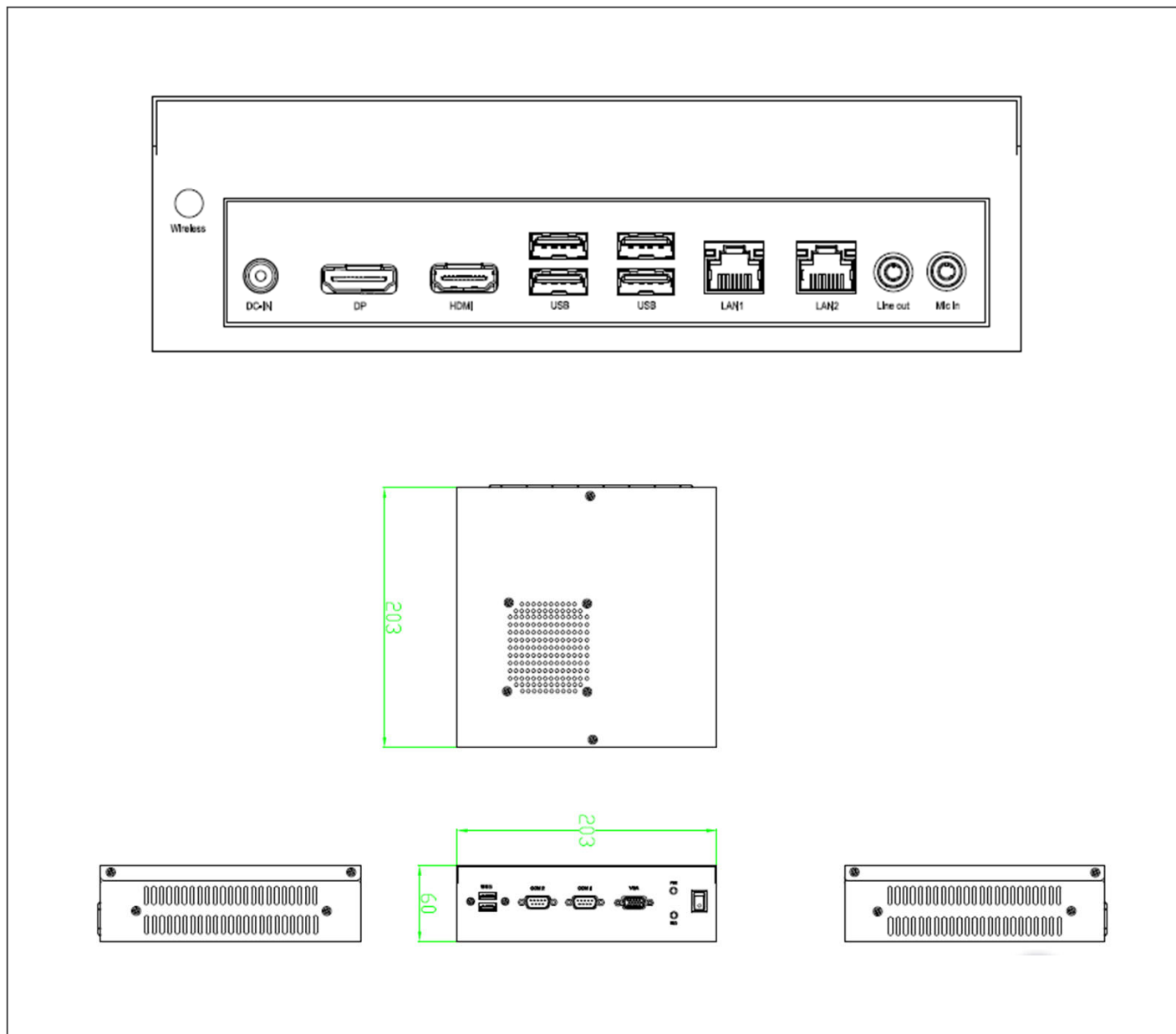
接口尺寸图 (单位: mm)
