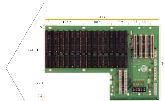
BP-219SG-P4-V60 > Segments : 1 Segment > Slot : 2 x PICMG , 4 x PCI , 13 x ISA > Chassis : ARC-6620
