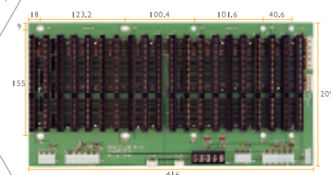
BP-220DI-V60 > Segments : 2 Segment > Slot : 20 x ISA > Chassis : ARC-6620
