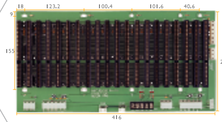
BP-220SI-V60 > Segments : 1 Segment > Slot : 20 x ISA > Chassis : ARC-6620
