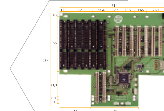
BP-214SG-P7-V22 > Segments : 1 Segment > Slot : 2 x PICMG , 7 x PCI , 5 x ISA > Chassis : ARC-6414
