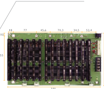
BP-214DI-V60 > Segments : 2 Segment > Slot : 14 x ISA > Chassis : ARC-6414
