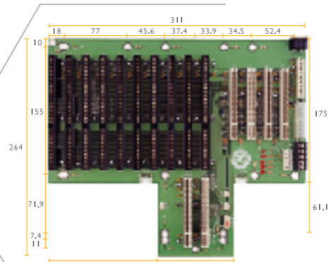
BP-214SG-P4-V65 > Segments : 1 Segment > Slot : 2 x PICMG , 4 X PCI , 8 x ISA > Chassis : ARC-6414
