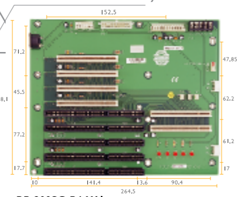
BP-209SG-P4-V61 > Segments : 1 Segment > Slot : 2 x PICMG , 4 x PCI , 3 x ISA
