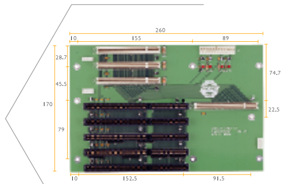
BP-208SG-P3-A10 > Segments : 1 Segment > Slot : 1 x PICMG , 3 X PCI , 4 x ISA
