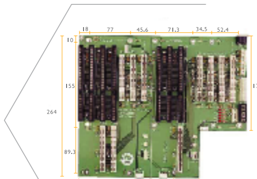
BP-213DG-P6-V60 > Segments : 2 Segments > Slot : 3 x PICMG , 7 x PCI , 4 x ISA > Chassis : ARC-6414
