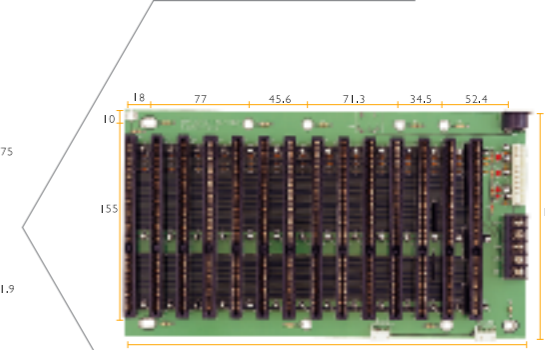
BP-214SI-V61 > Segments : 1 Segment > Slot : 14 x ISA > Chassis : ARC-6414
