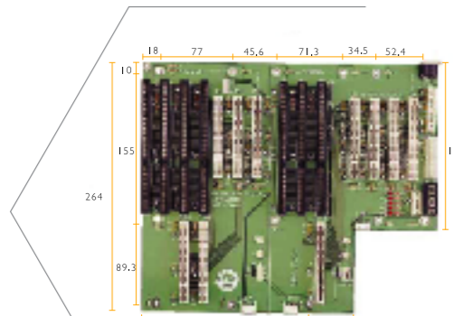
BP-212DG-P6-V61 > Segments : 2 Segments > Slot : 3 x PICMG , 7 x PCI , 4 x ISA > Chassis : ARC-6414
