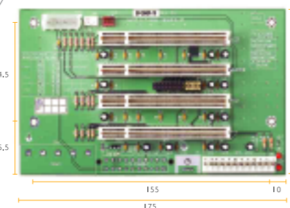
BP-204SP-A10 > Segments : 1 Segment > Slot : 1 x PICMG , 3 X PCI > Chassis : AEC-204
