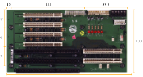
BP-206SG-P3-V61 > Segments : 1 Segment > Slot : 2 x PICMG , 4 X PCI , 1 x ISA > Chassis : AEC-206
