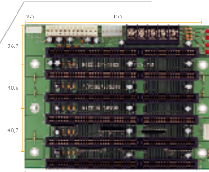
BP-206SI-V60 > Segments : 1 Segment > Slot : 6 x ISA > Chassis : AEC-206
